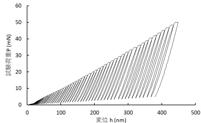
《荷重変位曲線》
