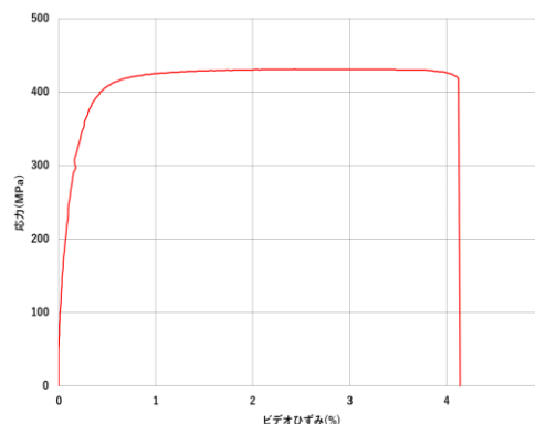
〈 応力－ビデオひずみ線図 (150℃) 〉
